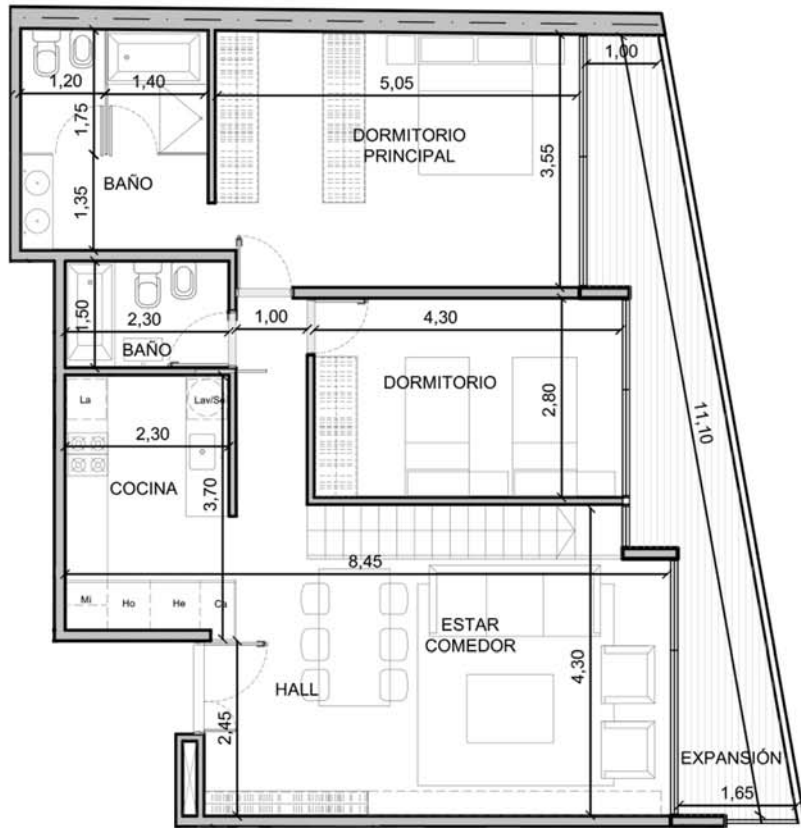
PLANTA BAJA
