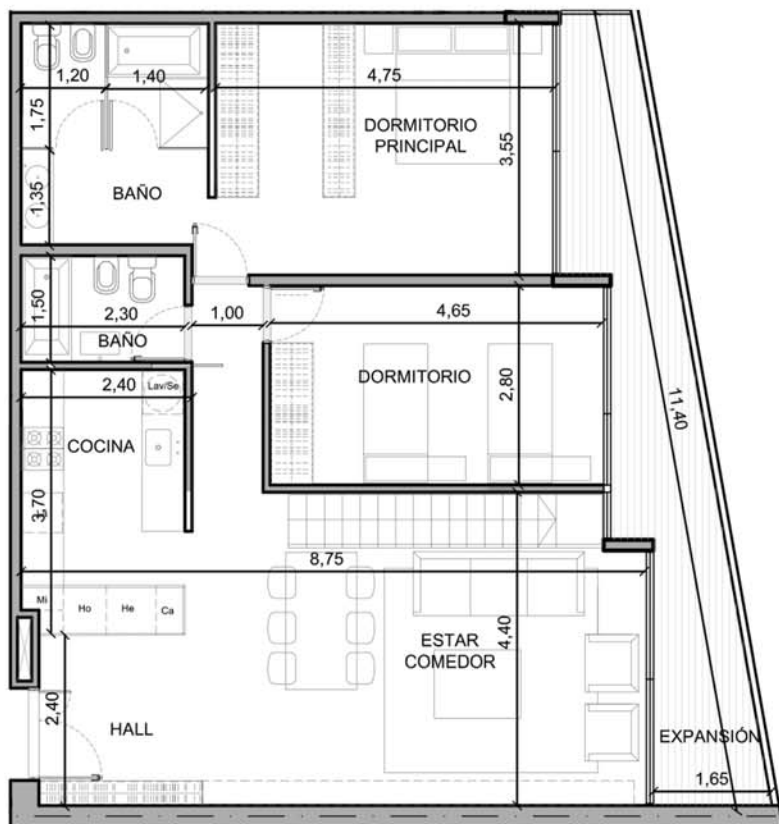
PLANTA BAJA
